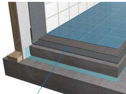
PROFAB BP membrane
